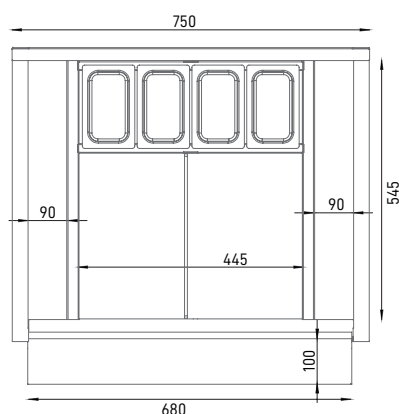
WHS 75 LATO / SIDE
