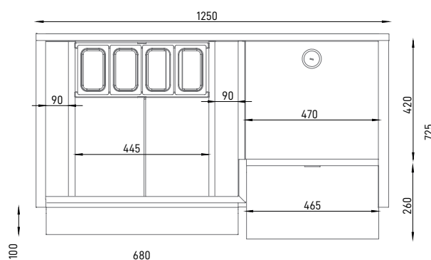
WHS 125 LATO / SIDE
