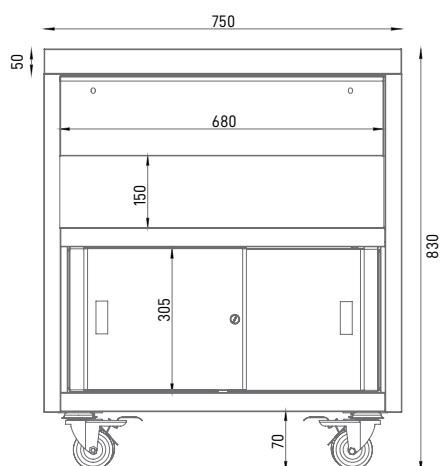
WHS 75 FRONTE / FRONT
