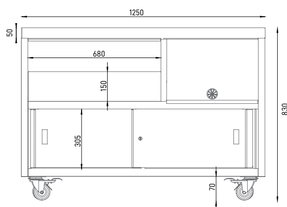
WHS 125 FRONTE / FRONT
